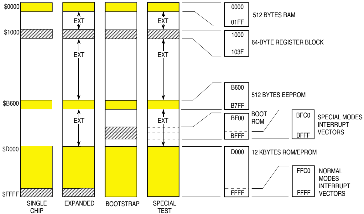
EA9 MEM MAP
