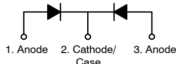
Schottky Diode
