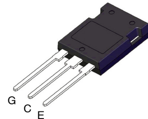
TO-247-3LD CASE 340CD
