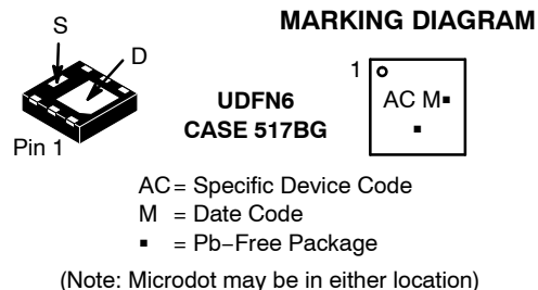
P-Channel MOSFET
