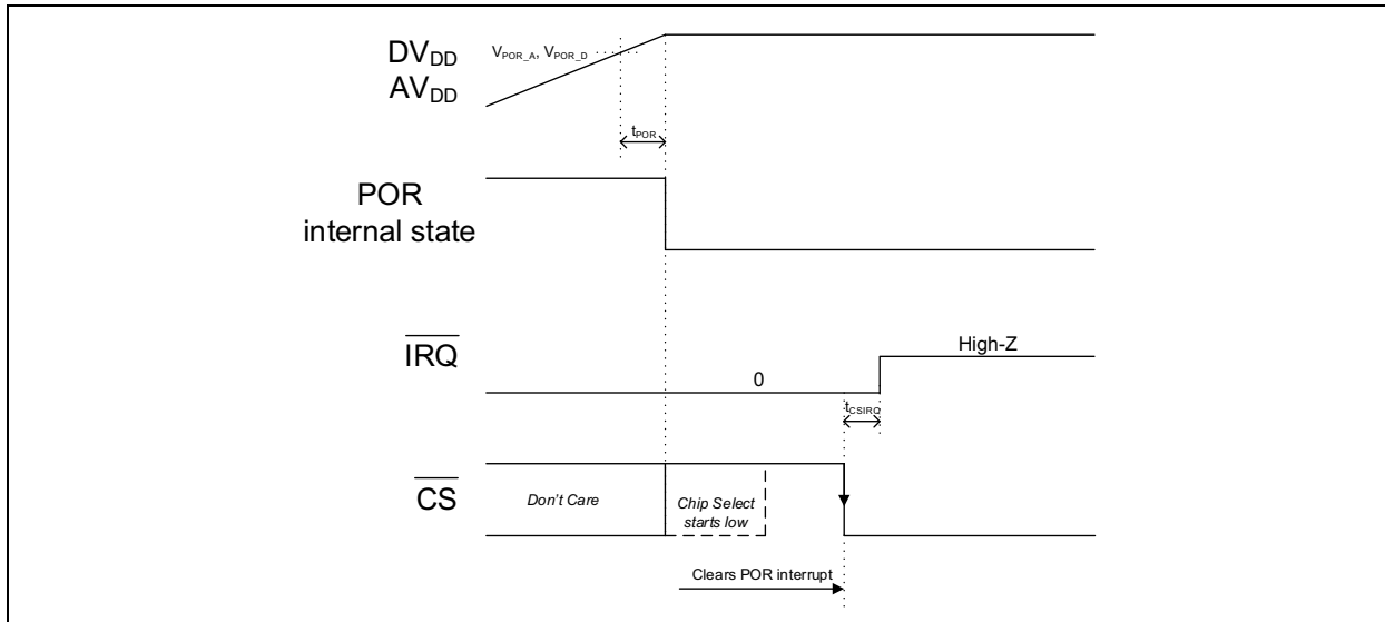
FIGURE 6-15: POR IRQ Timing Diagram.
